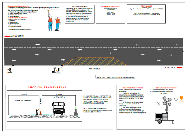
PLANO DE SENALAMIENTO DE PROTECCIÓN DE OBRA PARA EL CONFINAMIENTO DE UN CARRIL Y ACOTAMIENTO DE LA AUTOPISTA TOLUCA-ZITÁCUARO PARA CONSTRUCCIÓN DE FILTRO EN EL KM 105+800
